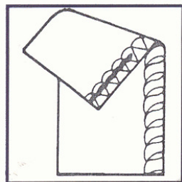
Exemple sur surjeteuse 1-aiguille
